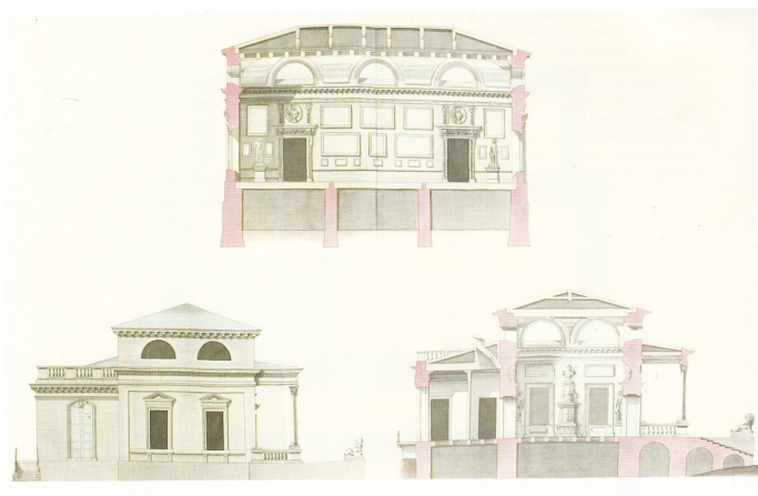
Проект Картинной галереи (фасад, разрез) архитектора В. И. Баженова
