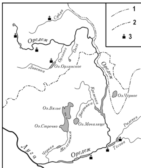
Бассейн р. Оредеж: 1 — границы летописной Ижорской земли (по Е.А. Рябинину); 2 — уездные границы XV–XVIII вв.; 3 — центры погостов XV в.
