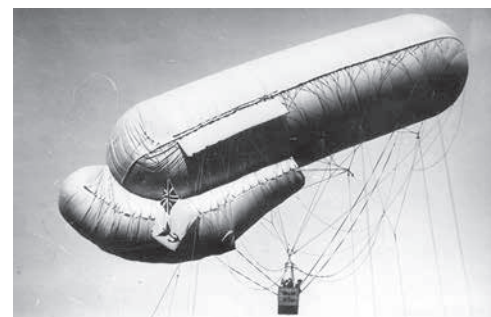
Змейковый аэростат (привязной) на воздухоплавательном полигоне в деревне Сализи. Фото 1912 года
